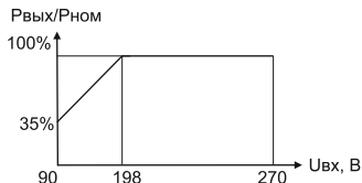
Рисунок 1. Зависимость выходной мощности от входного напряжения, где U_{\text{вх}} – входное напряжение, R_{\text{вых}} – выходная мощность, R_{\text{ном}} – номинальная (паспортная) выходная мощность.
